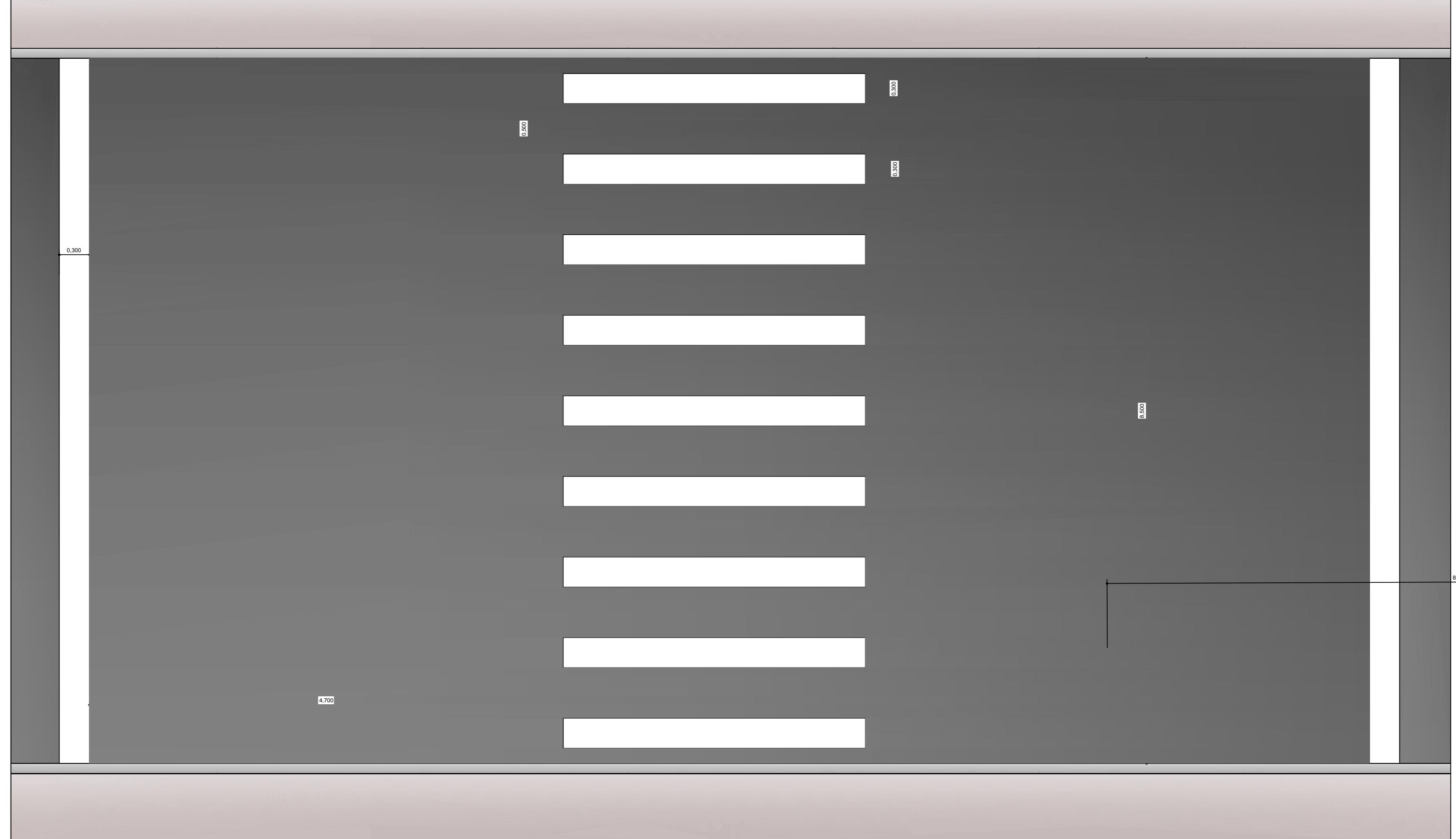
DETALHE EM VISTA SUPERIOR DA SINALIZAÇÃO HORIZONTAL PARA ACESSIBILIDADE EM FRENTE AO REBAIXAMENTO DO PASSEIO ESCALA : 1 / 30
