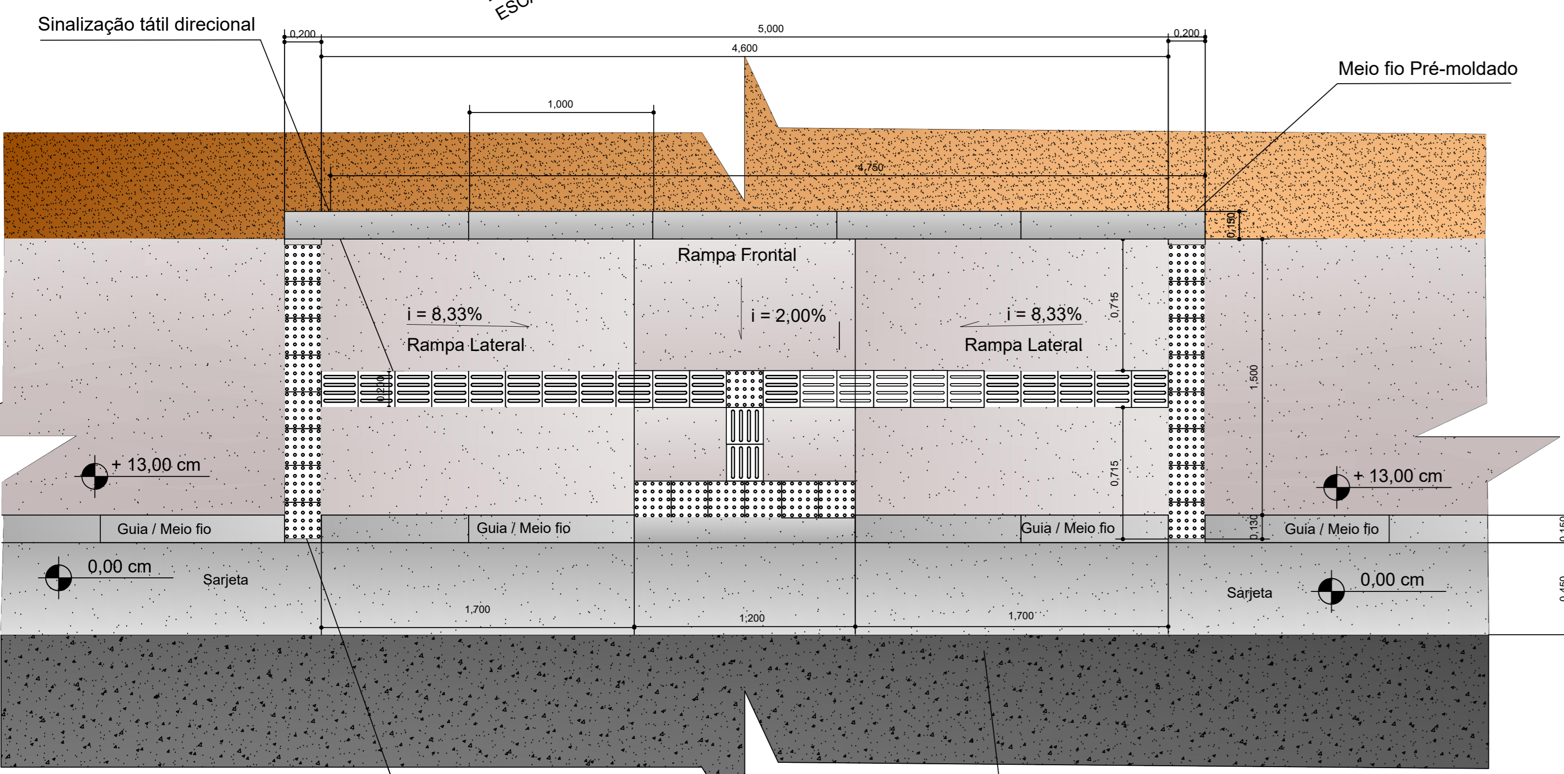
DETALHE EM VISTA SUPERIOR DO REBAIXAMENTO PARA ACESSIBILIDADE DO PASSEIO (CALÇADA) ESCALA : 1 / 20
