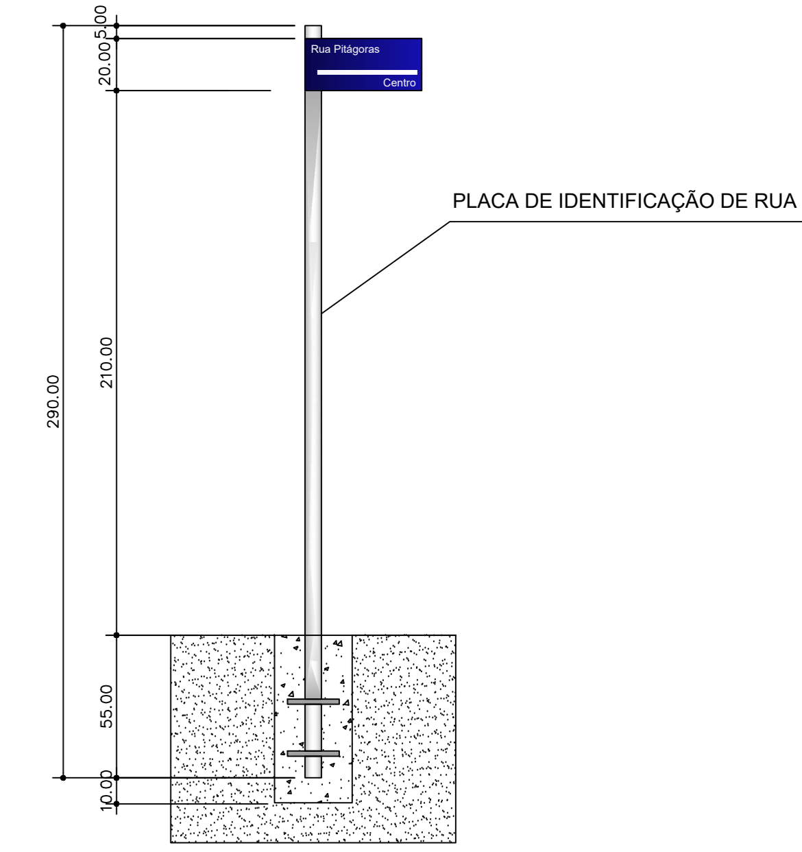
DETALHE PLACA DE IDENTIFICAÇÃO DE RUA SEM ESCALA
