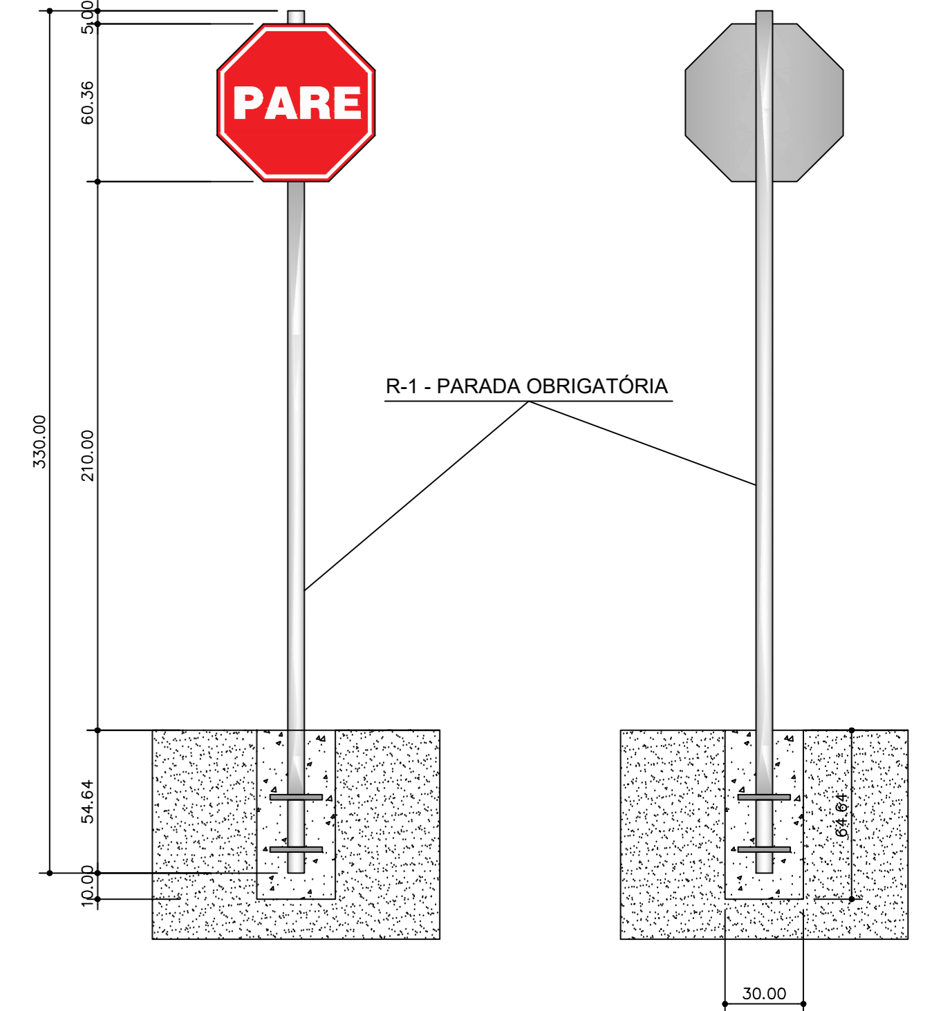
DETALHE PLACA DE REGULAMENTAÇÃO R-1 SEM ESCALA
